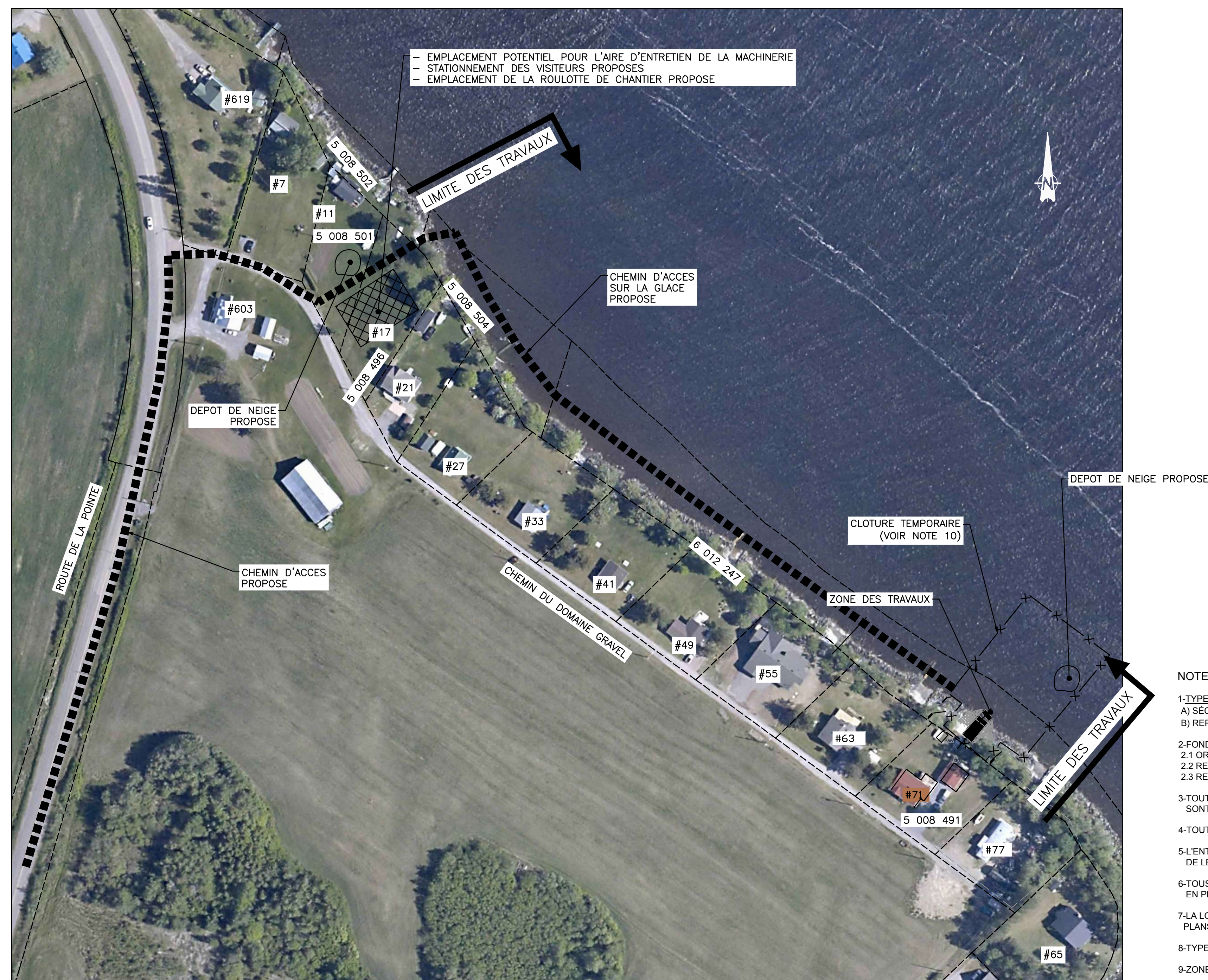
VUE EN PLAN EMPLACEMENT DE L'AIRE D'ENTRETIEN DE LA MACHINERIE ET CHEMIN D'ACCES PROPOSE ECHELLE 1:1000
