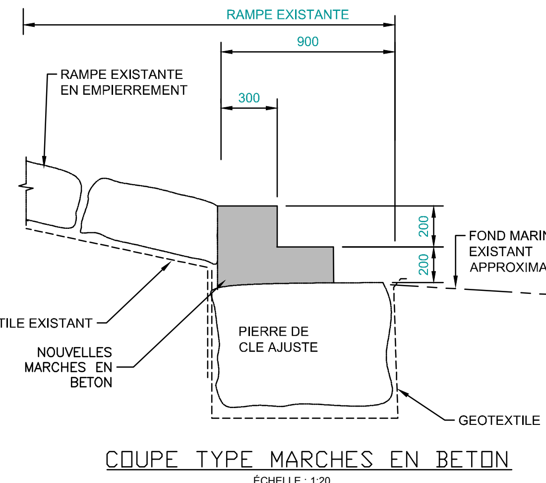
COUPE TYPE MARCHES EN BETON
