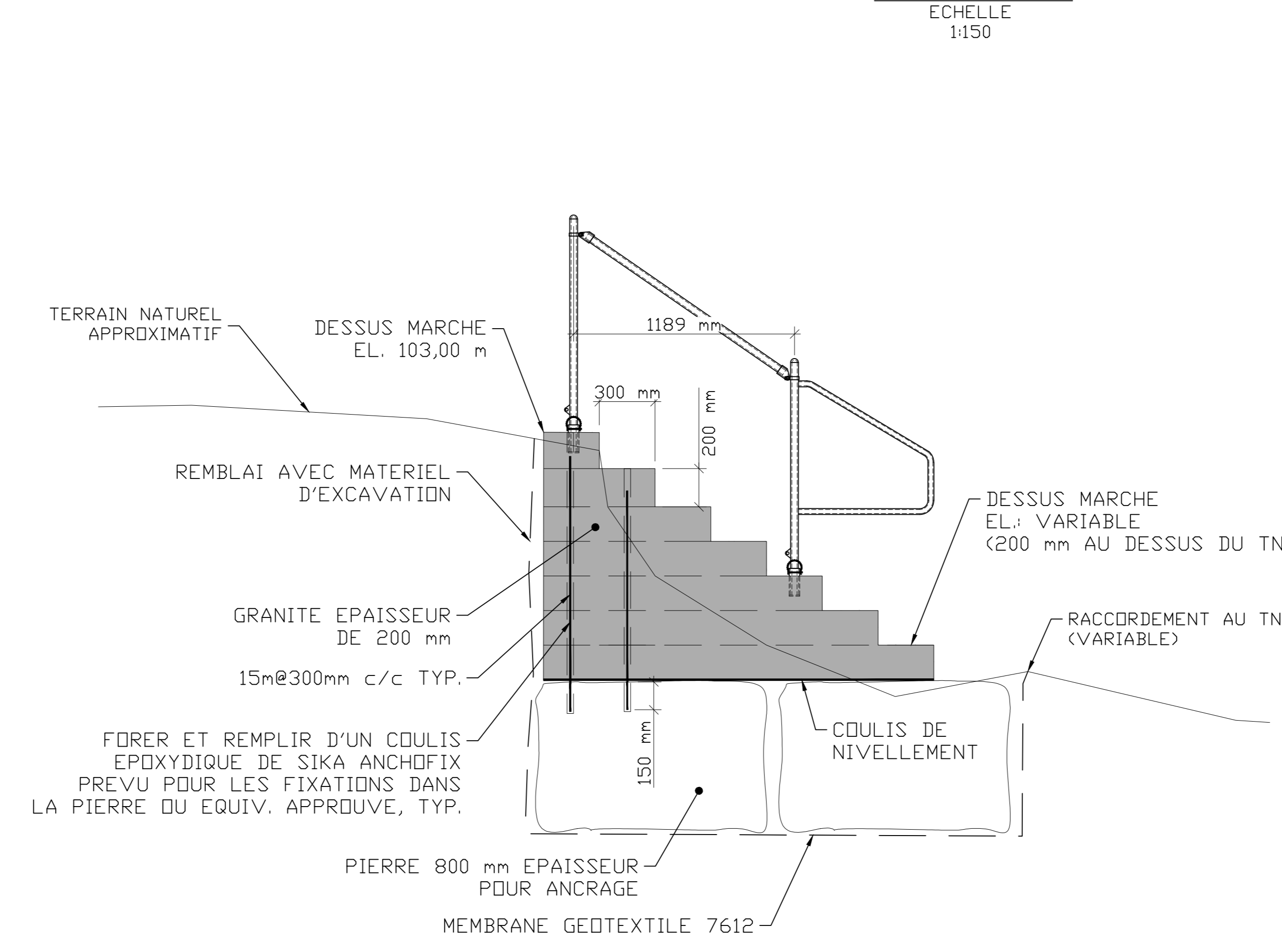
ESCALIER EN GRANIT AVEC GARDE-CORPS AMOVIBLE DETAIL TYPE Echelle: 1:20
