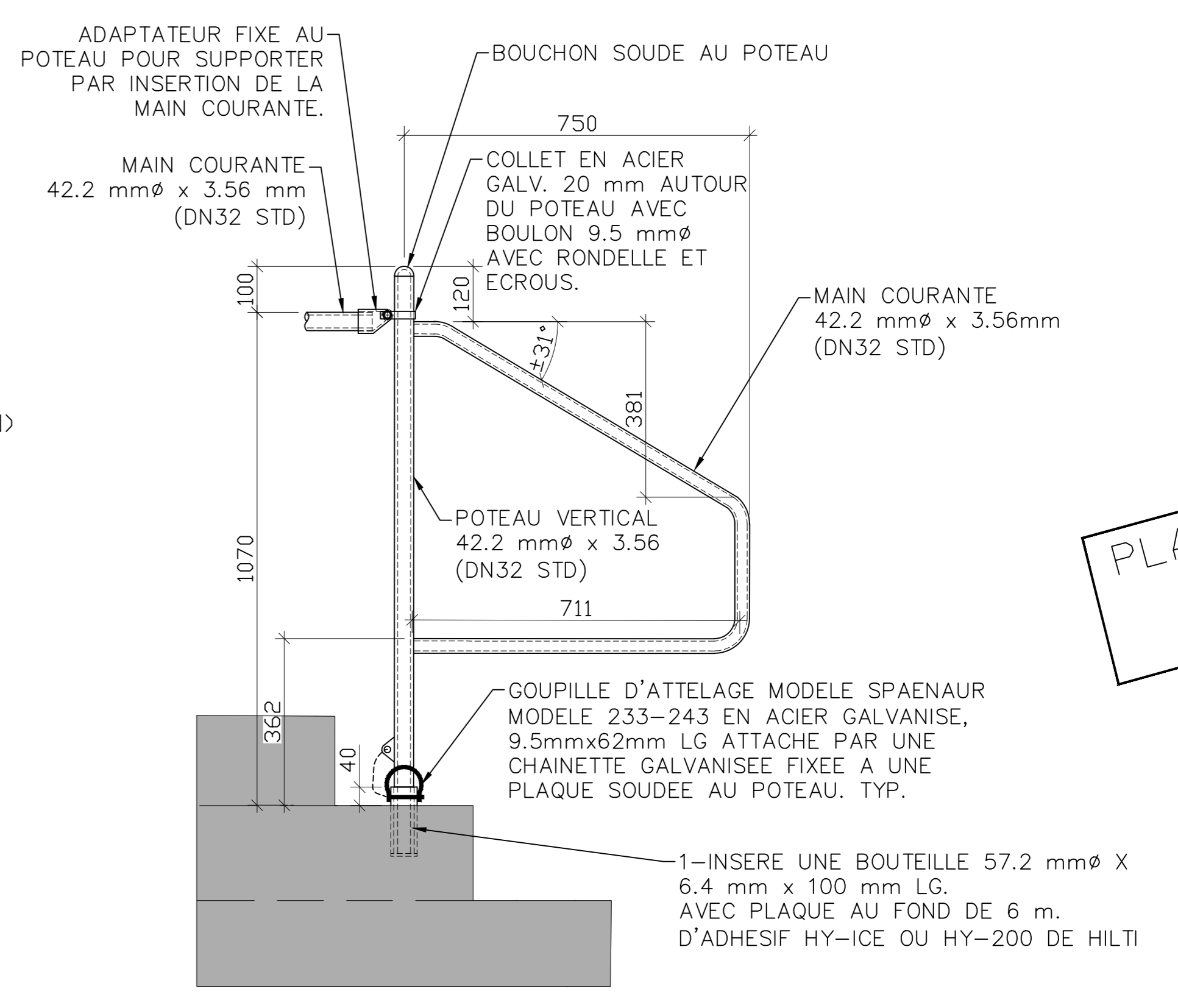
DETAIL EXTREMITÉ Echelle: N.A.E.
