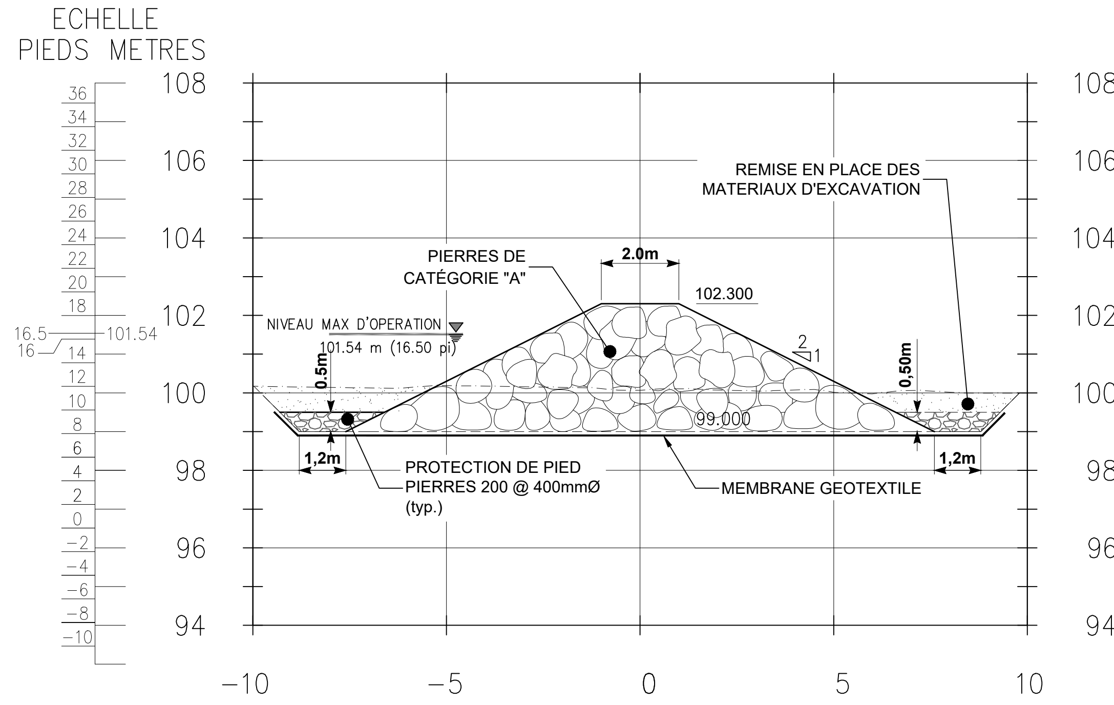
SECTION 6 H: 1:100 V: 1:100
