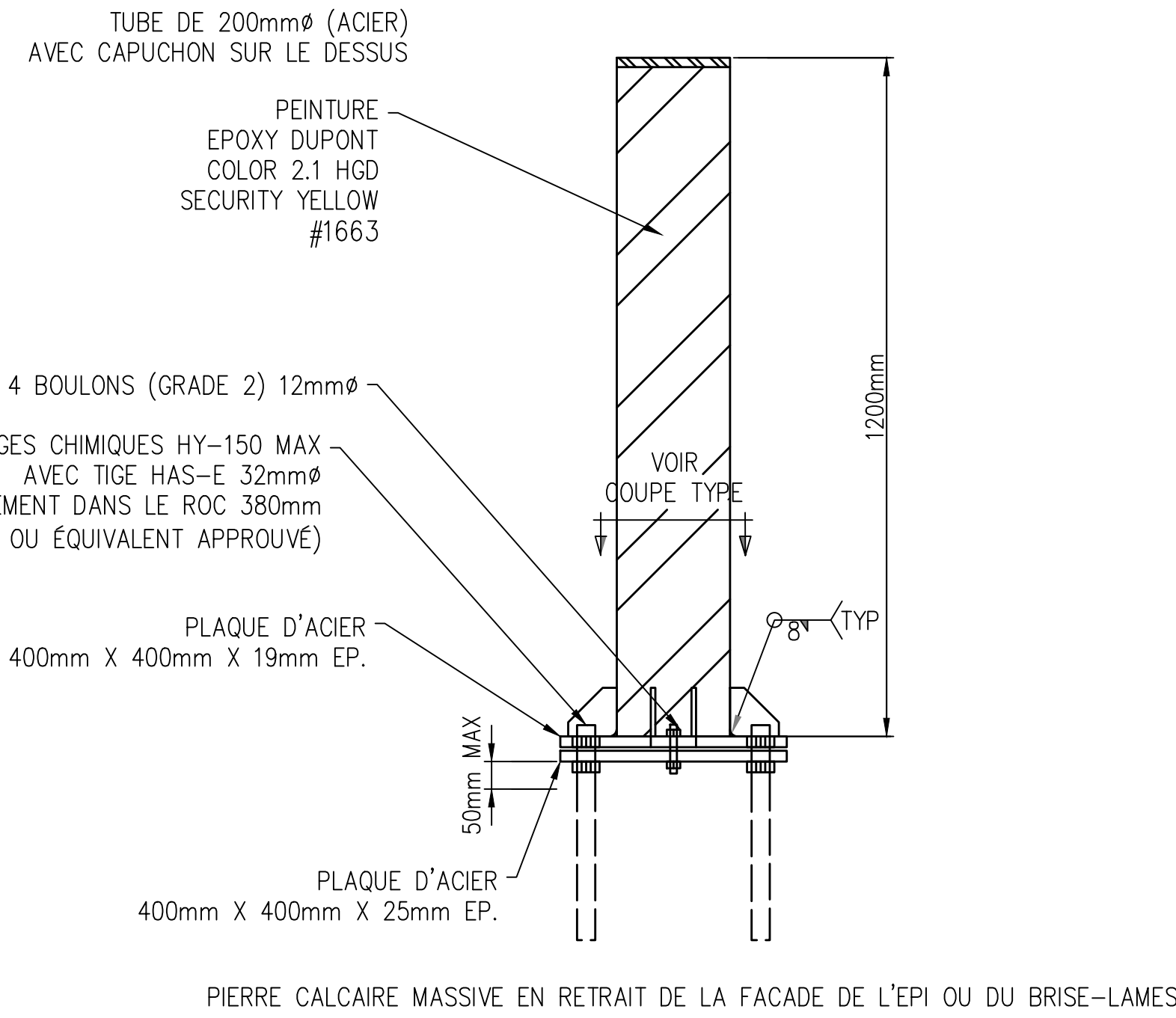
DETAIL DE BALISE D'AIDE A LA NAVIGATION ECH. 1:10
