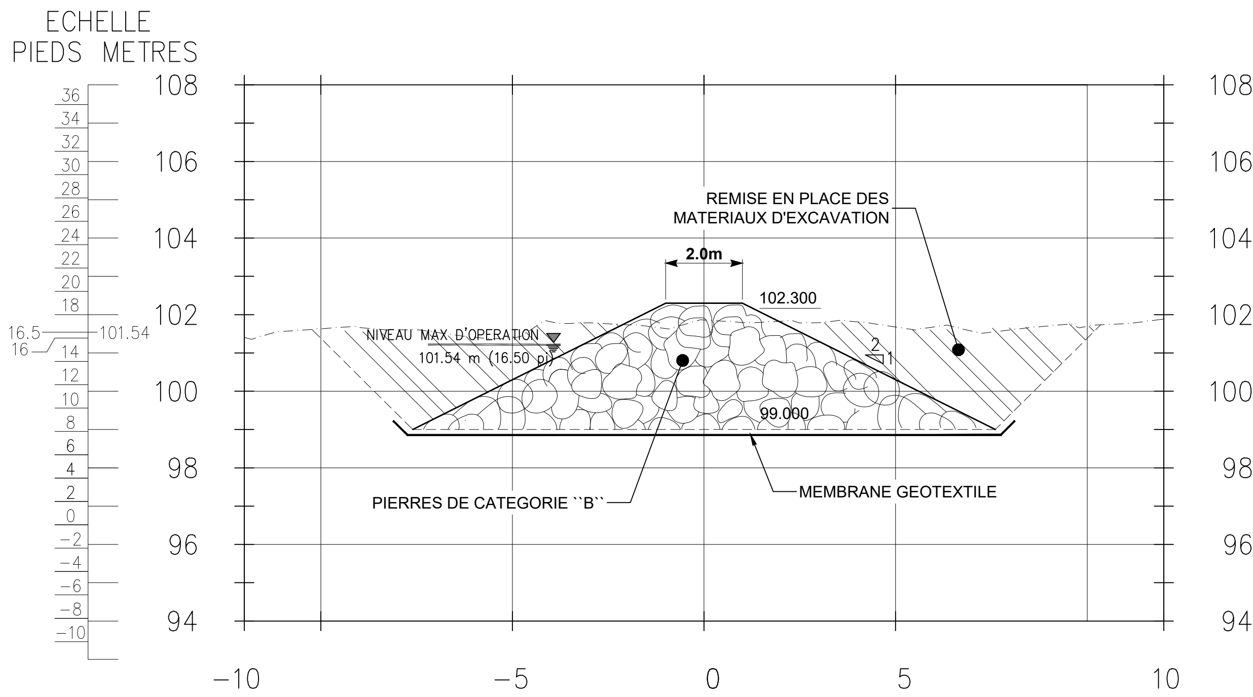
SECTION 4 H: 1:100 V: 1:100
